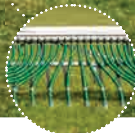
Gleichmäßige Verteilqualität durch kurze Auslaufschläuche
