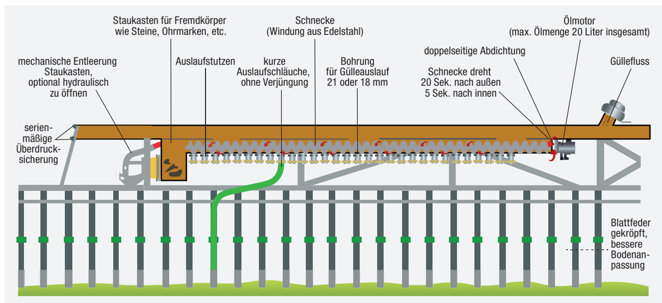
Bild 6: FLIEGL Schneckenverteiler
